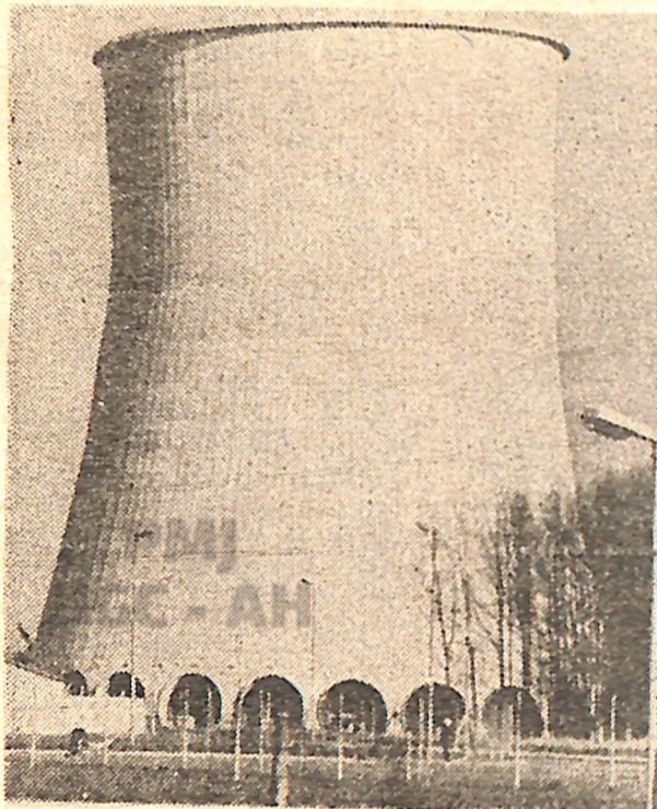
Refrigerador — com 80 metros de altura — é o responsável pelo resfriamento da água.
